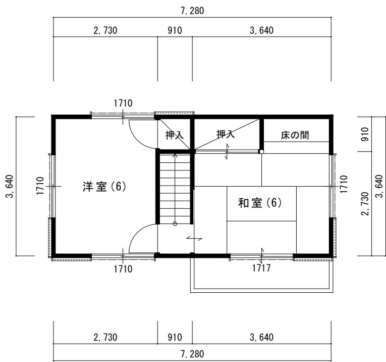
2階平面図 1 : 100
