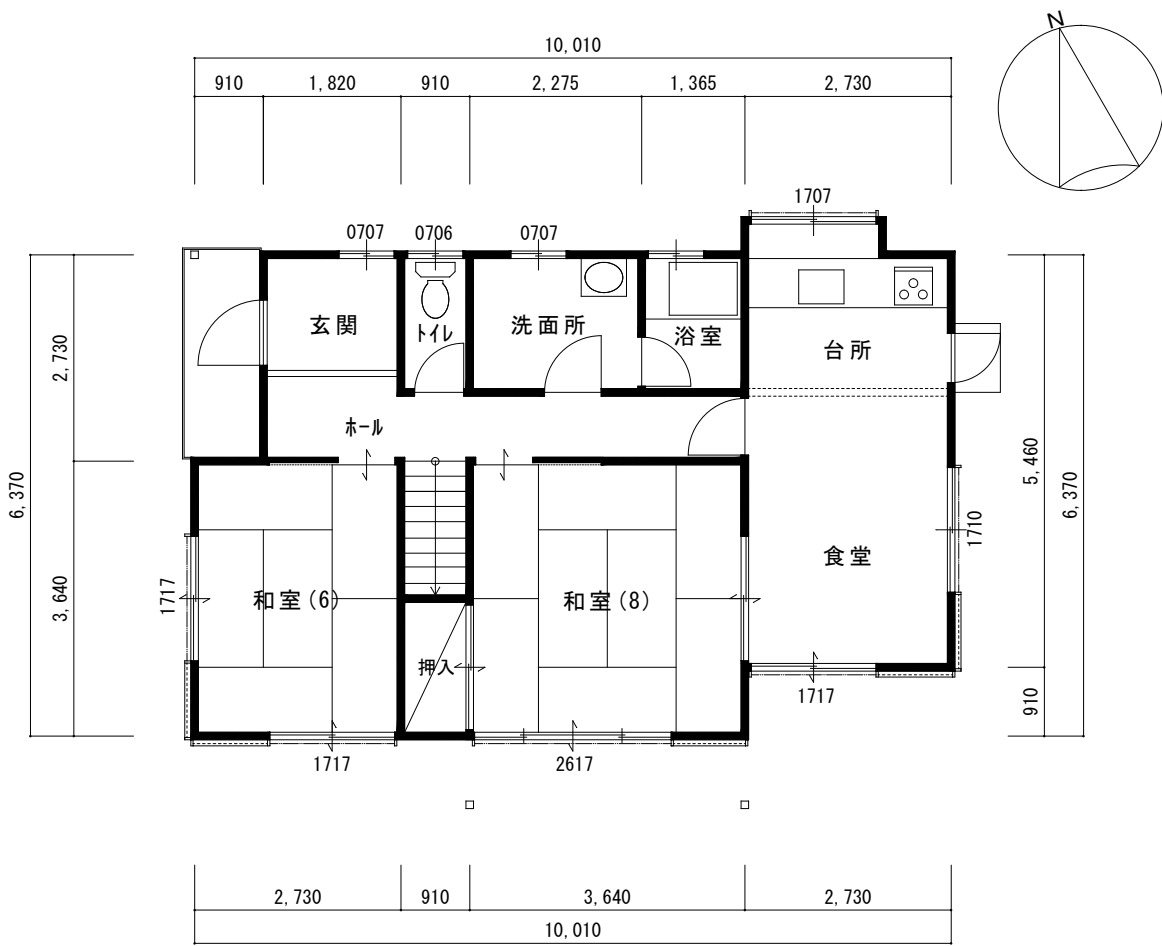
1階平面図 1 : 100
